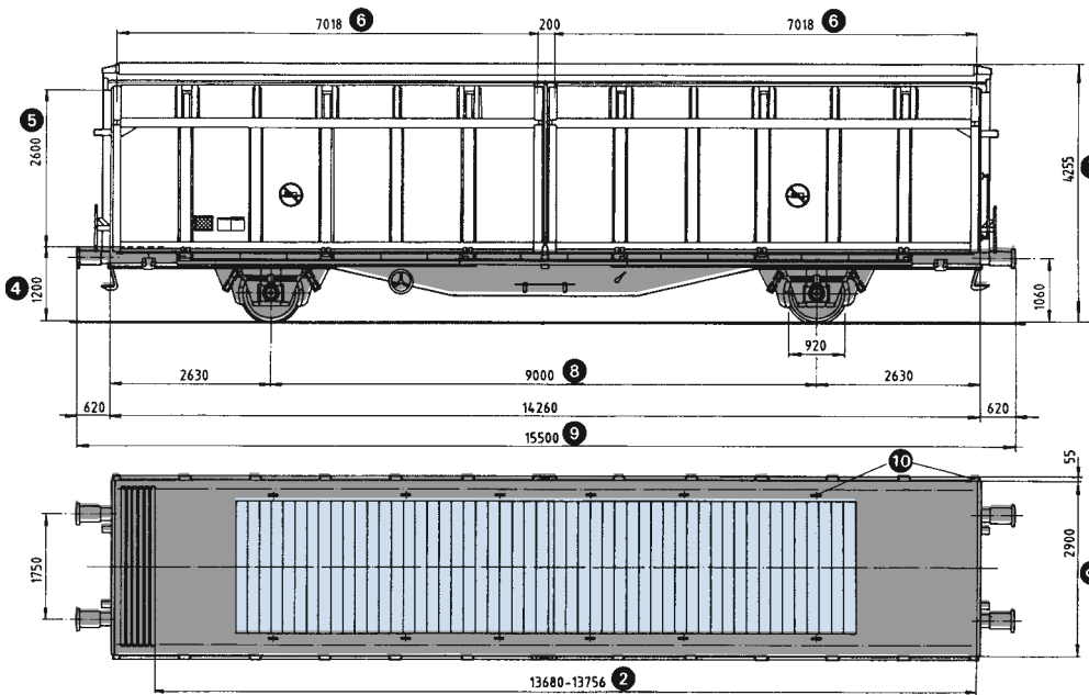
Longueur de chargement des charges concentrées (indication ne figurant pas sur le wagon)
