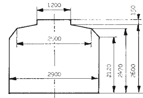
Vue en coupe du volume utile
